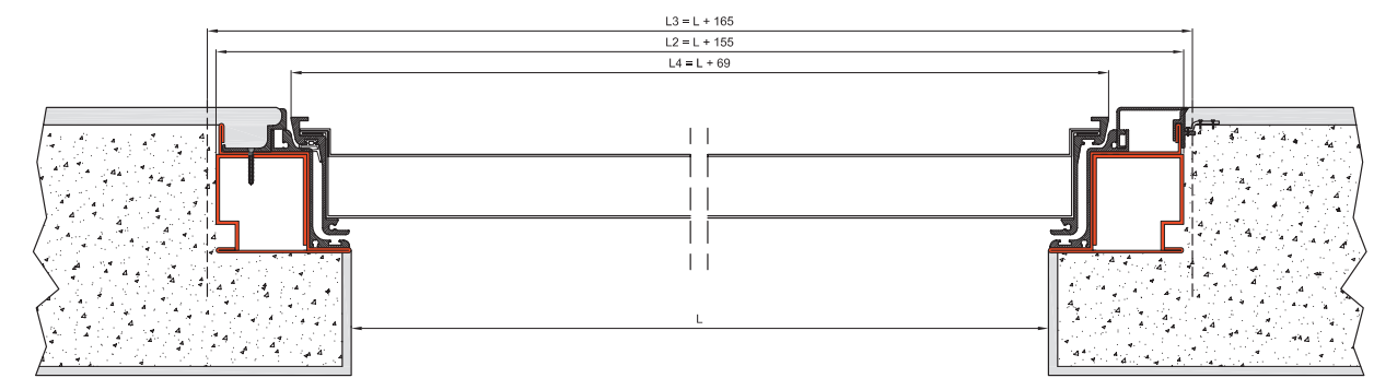
Soluzione 6 - Porta blindata filomuro per muratura Solution 6 - Armoured door flush with wall for masonry
