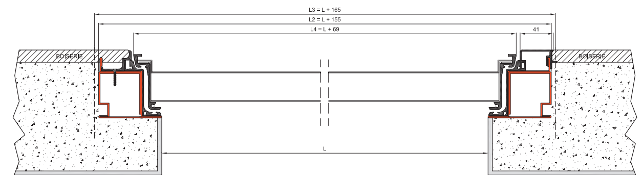
Soluzione 6 - Porta blindata a filomuro per boiserie Solution 6 - Armoured door flush with wall for panelling
