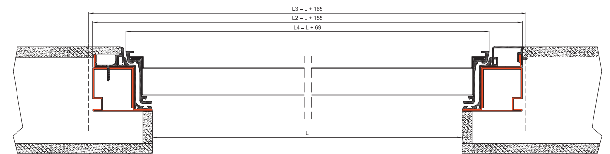
Soluzione 6 - Porta blindata a filomuro per cartongesso Solution 6 - Armoured door flush with wall for plasterboard
