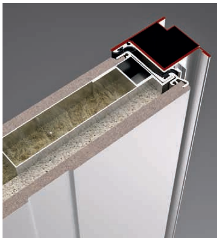
Pannello anta con spessore 14 mm, laccato 14 mm thick lacquered panel
