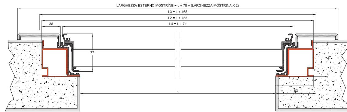
Soluzione 1 - Porta blindata a filo lato a tirare con mostrina Solution 1 - Armoured door flush on pull side with trim
