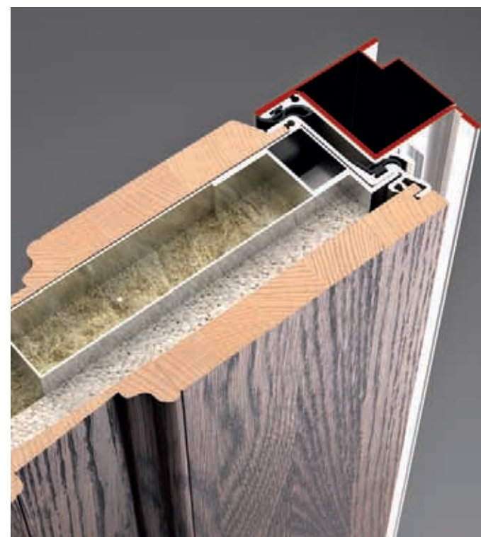
Pannello anta con spessore 22 mm, in legno massiccio 22 mm thick solid wood door panel
