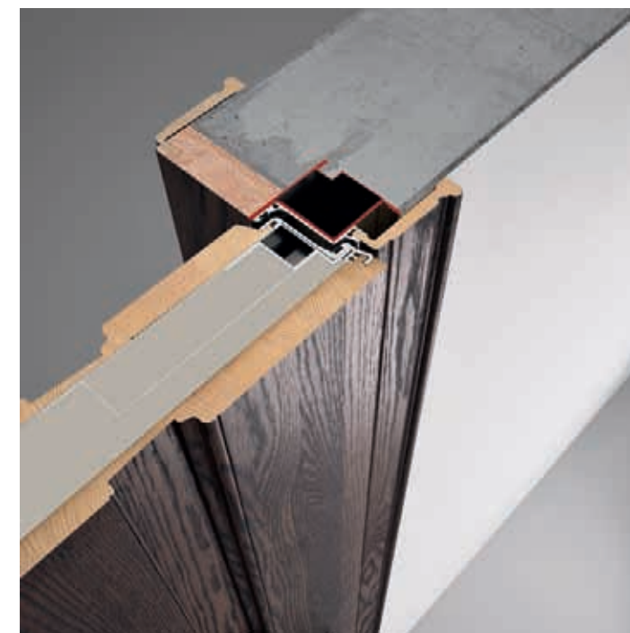
Soluzione 2 - Portone blindato a filo lato interno con mostrina, con imbotte in legno e mostrina lato esterno Solution 2 - Interior side security door with trim, with wood door jamb and exterior side trim
