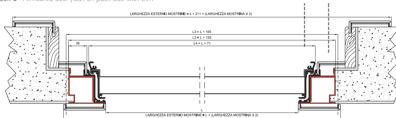
Soluzione 4 - Porta blindata a filo lato a spingere con mostrina e imbotte Solution 4 - Armoured door flush on push side with trim and intrados
