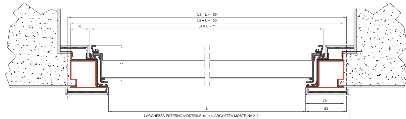
Soluzione 3 - Porta blindata a filo lato a spingere con mostrina Solution 3 - Armoured door flush on push side with trim
