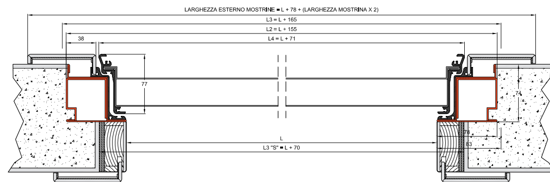
Soluzione 2 - Porta blindata a filo lato a tirare con mostrina e imbotte Solution 2 - Armoured door flush on pull side with trim and intrados
