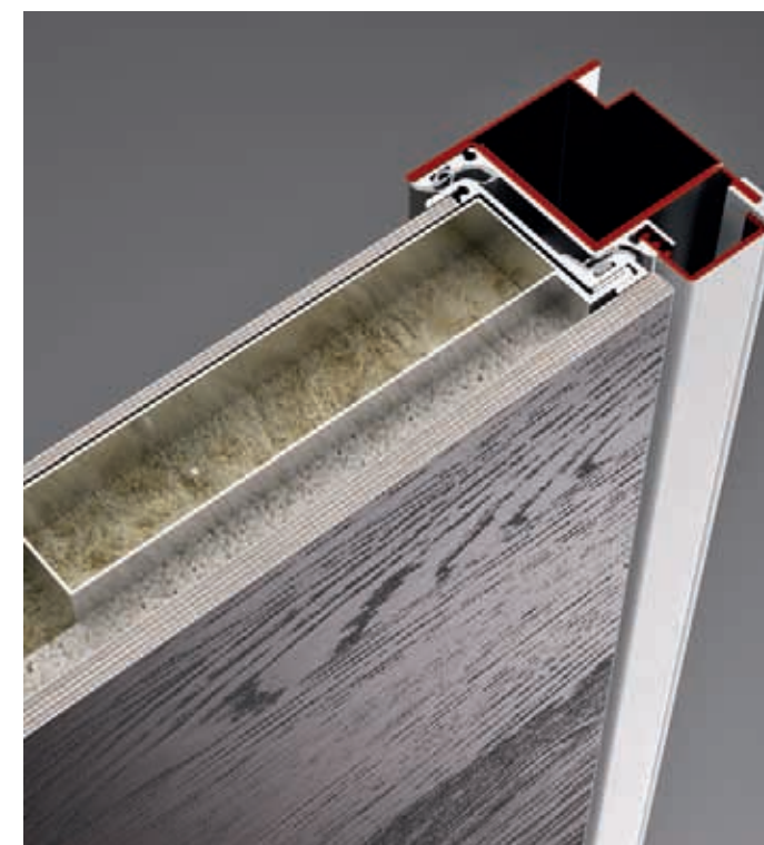
Pannello anta con spessore 12 mm tipologia Filomuro, laccato o impiallacciato legno 12 mm thick lacquered or veneered wood Filomuro door panel
