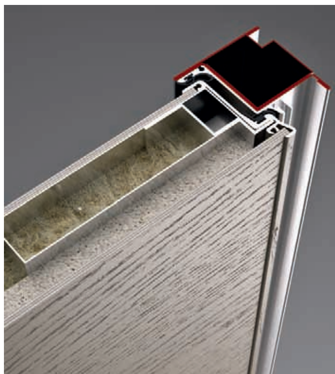
Pannello anta con spessore 6 mm, laccato o impiallacciato legno 6 mm thick lacquered or veneered wood door panel
