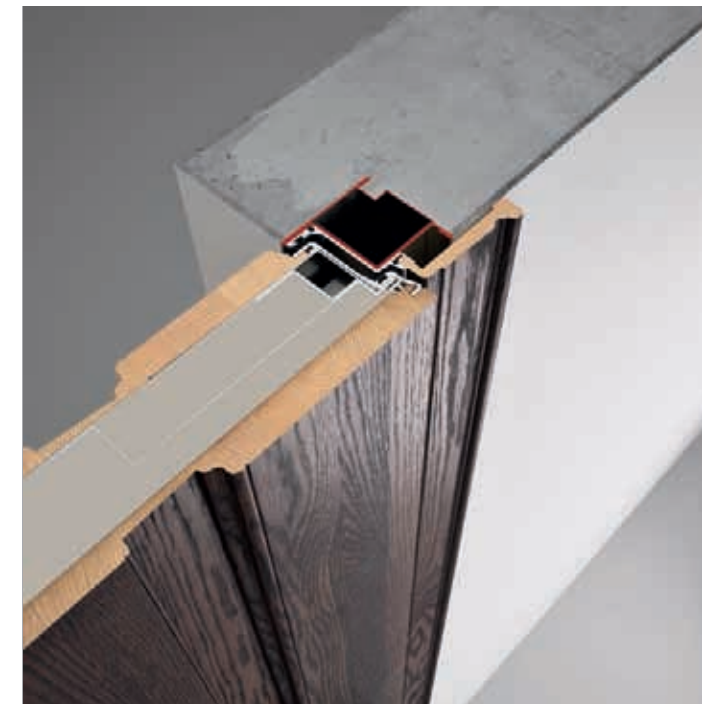
Soluzione 1 - Portone blindato a filo lato interno con mostrina Solution 1 - Interior side security door with trim
